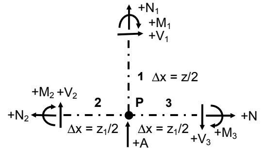
Fig. 3.3a Nomenclatura empleada para designar los esfuerzos. La dirección de las flechas indica el valor positivo.
