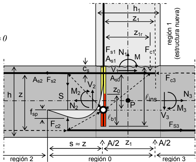
Fig. 3.3c Nudo pórtico con modelo de bielas y tirantes
