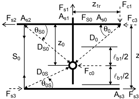
Fig. 3.3b Modelo de bielas y tirantes Limitación: 0.58 \leq \cot \theta_1 \leq 2.0
